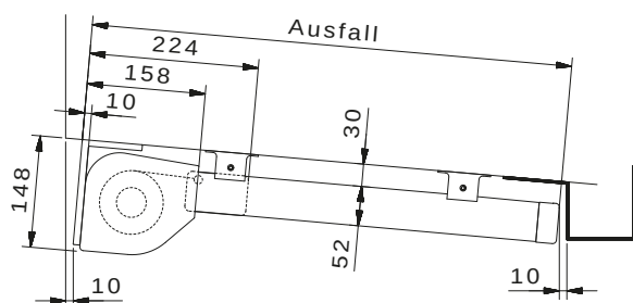
T200 Seitenansicht
