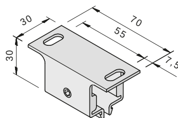
T90 Führungsschienenhalter
