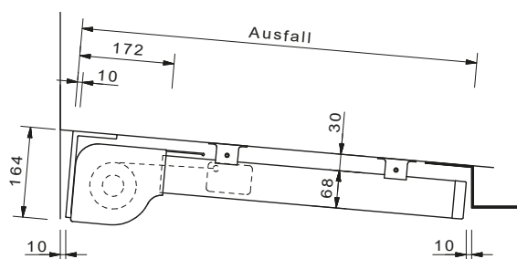
T200 Seitenansicht
