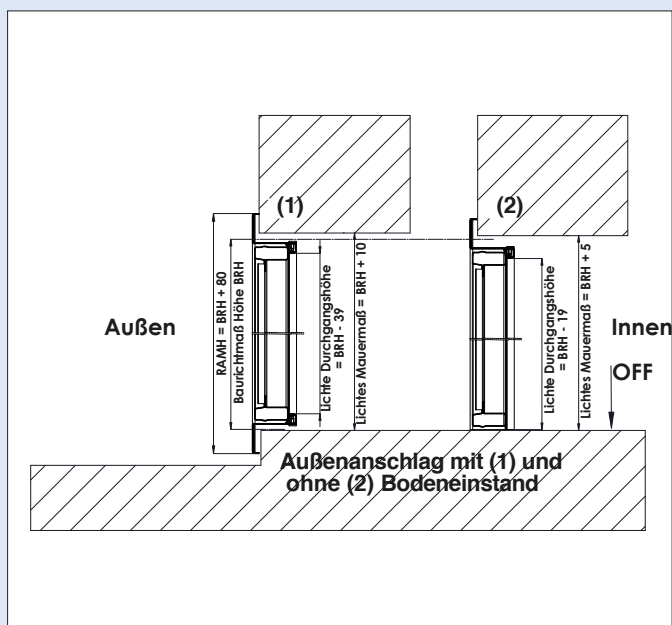
Anschlagarten
