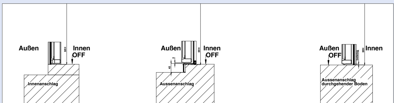
Anschlagarten
