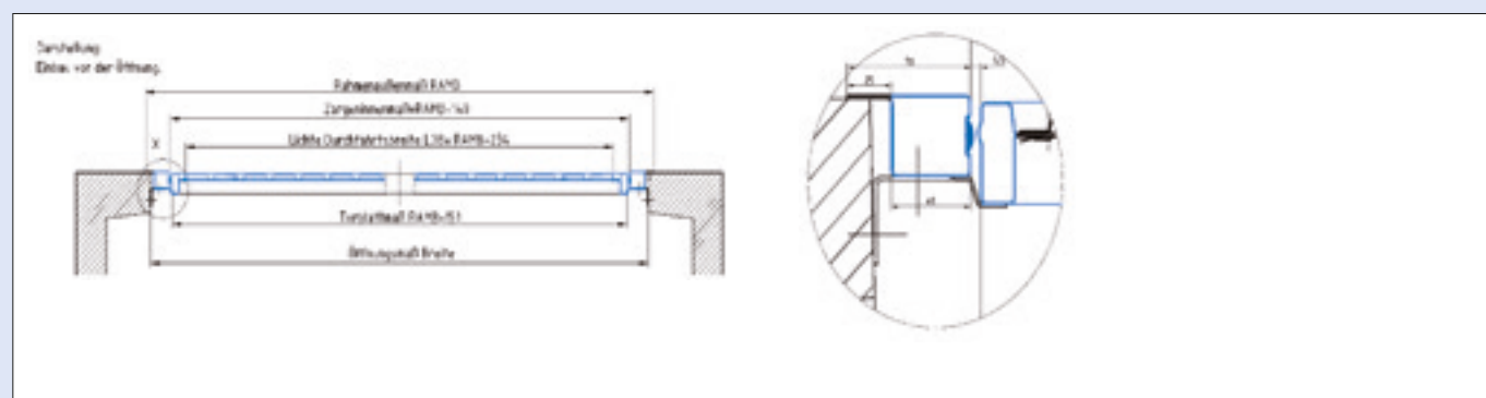
Typ Rees (Außenanschlag) - Horizontaler Torschnitt
