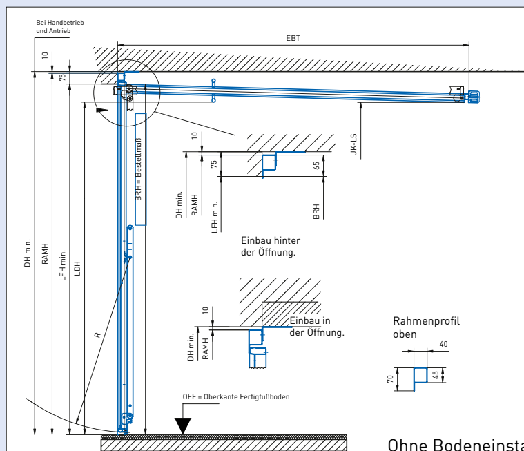
Mit Bodeneinstand
