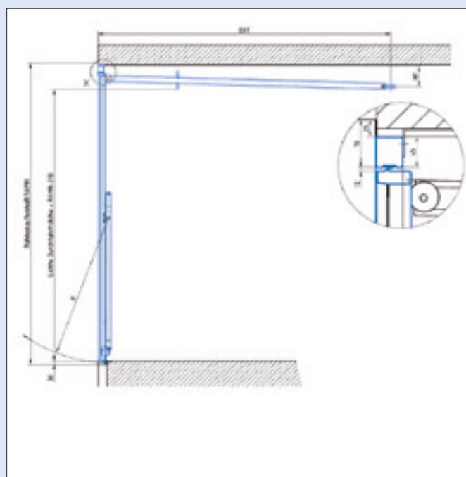
Typ Rees (Außenanschlag) - Vertikaler Torschnitt
