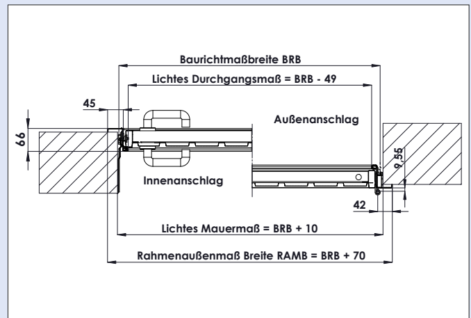
Einbau bei Innenanschlag
