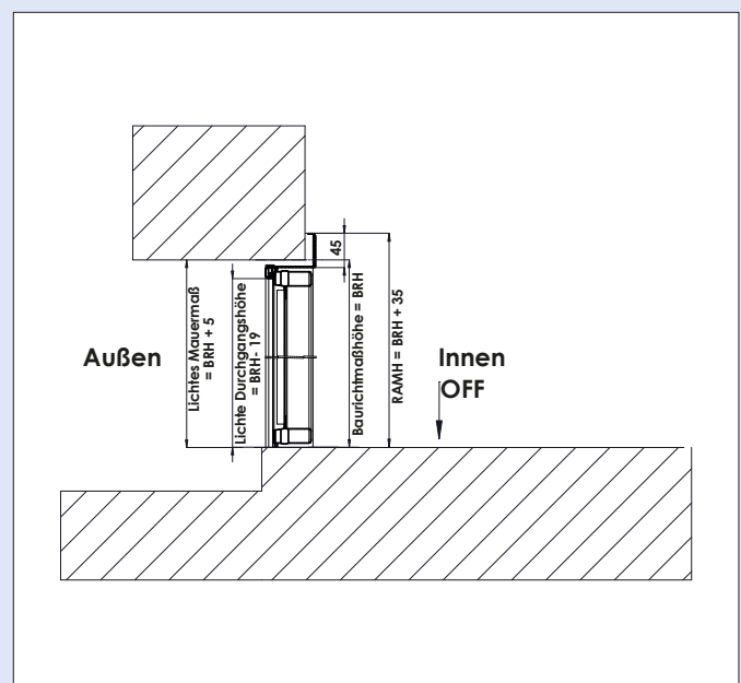
Einbau bei Innenanschlag
